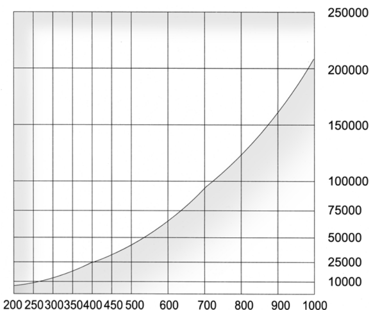
График зависимости DN-CV шиберной задвижки с перенаправляющим отверстием DN-CV Graph of Flat Valves with a Diversion Hole
